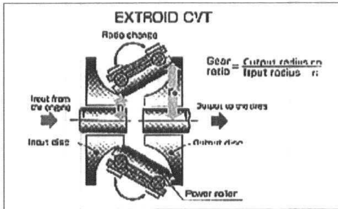
〈그림 2〉 Nissan Extroid CVT
